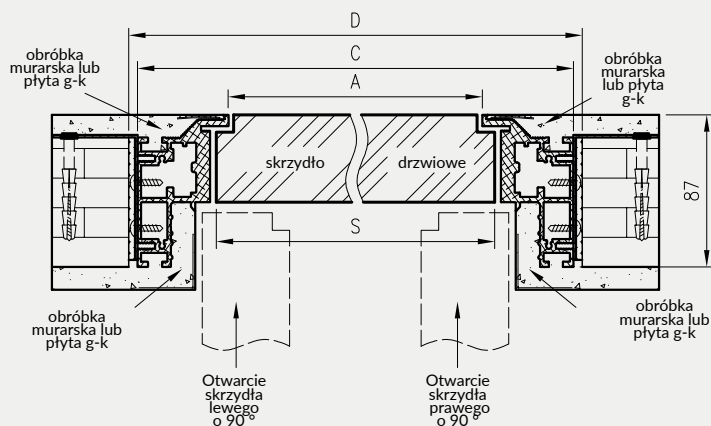
Przekrój poprzeczny drzwi 50mm z odwróconą przylgą - otwierane do wewnątrz
