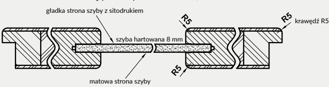
Przekrój poziomy drzwi VETRO A5, A10-A11
