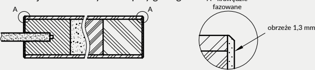
Przekrój ramienia skrzydła bezprzylgowego
