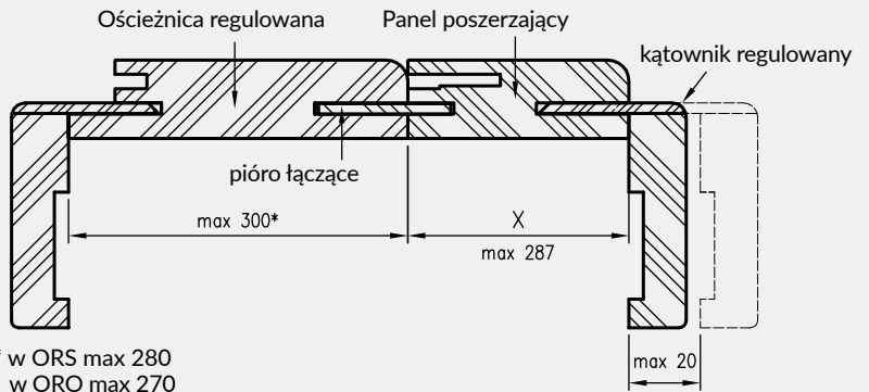
warianty szerokości przekroju panela
