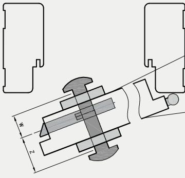
Rys. Dobór wymiaru wkładki z gałką
