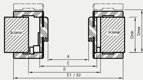
Przekrój poziomy ORB
